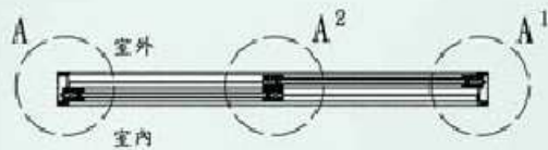
A-A' 水平剖面圖
