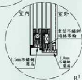
B¹ 大樣圖
