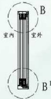
B-B' 垂直剖面圖
