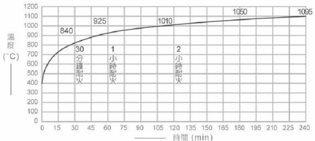
▲ 耐火標準加熱溫度-時間曲線圖
