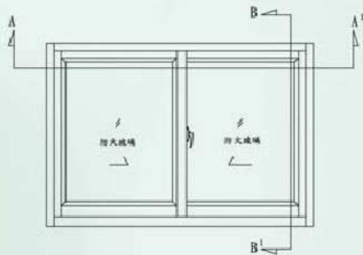
正立面圖(室內面)
